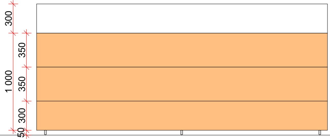
FRONT OPPRISS
