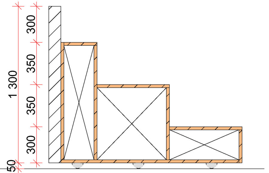
SNITT 1:20
