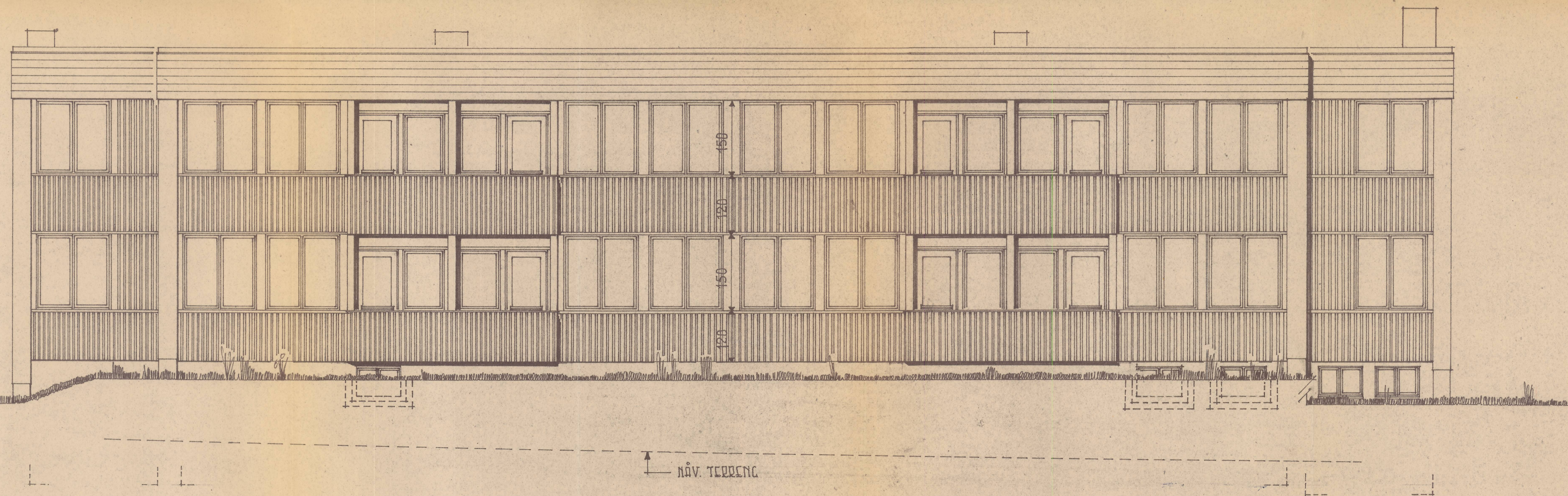
FASADE MOT ØST
