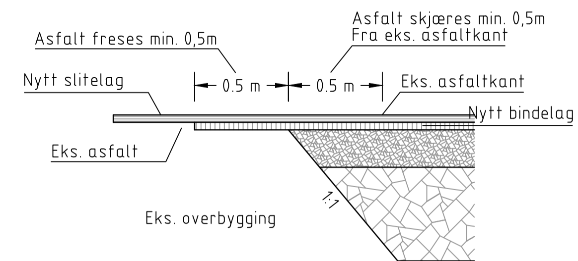
SPLEIS MOT EKS. VEI I SIDERETNING M=1:10
