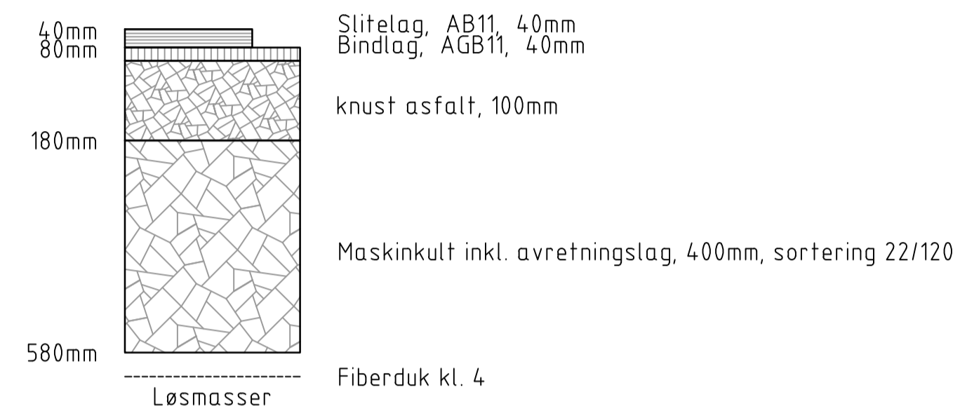
OVERBYGGING LØSMASSER TRAFFIKERT VEI M=1:10
