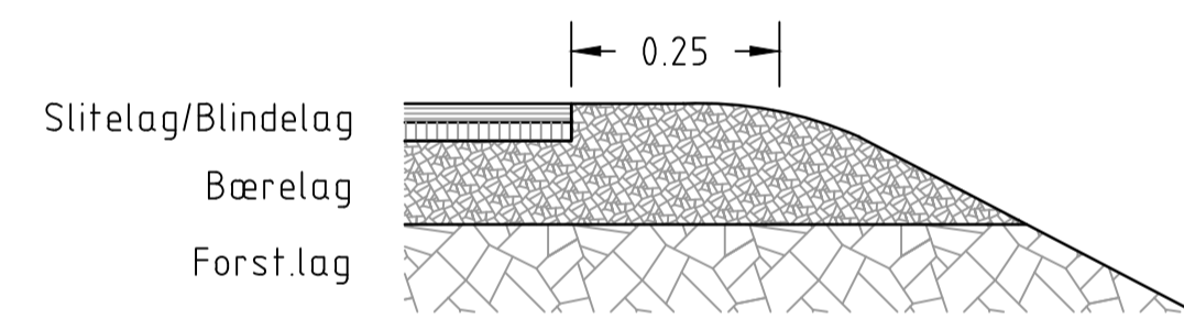
PRINSIPPSKISSE FOR UTFØRELSE AV SKULDER MOT GRØFT M=1:10
