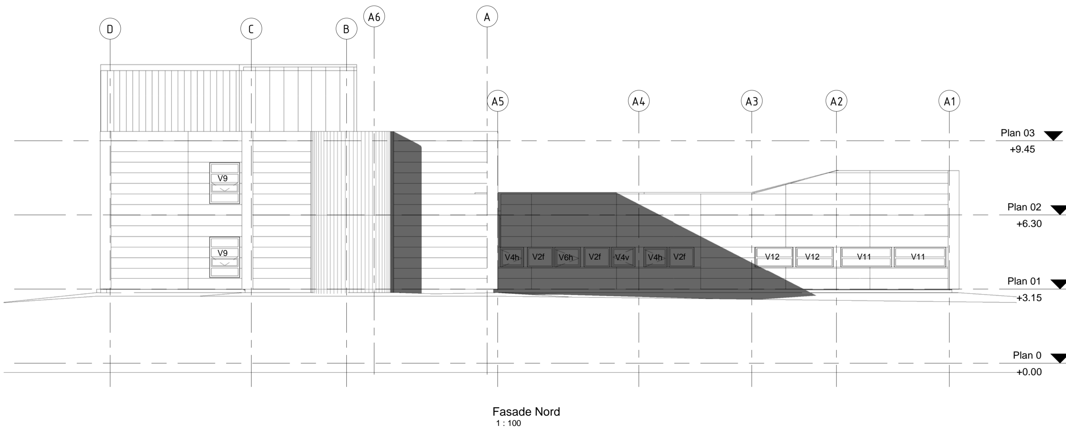
Fasade Vest 1 : 100
