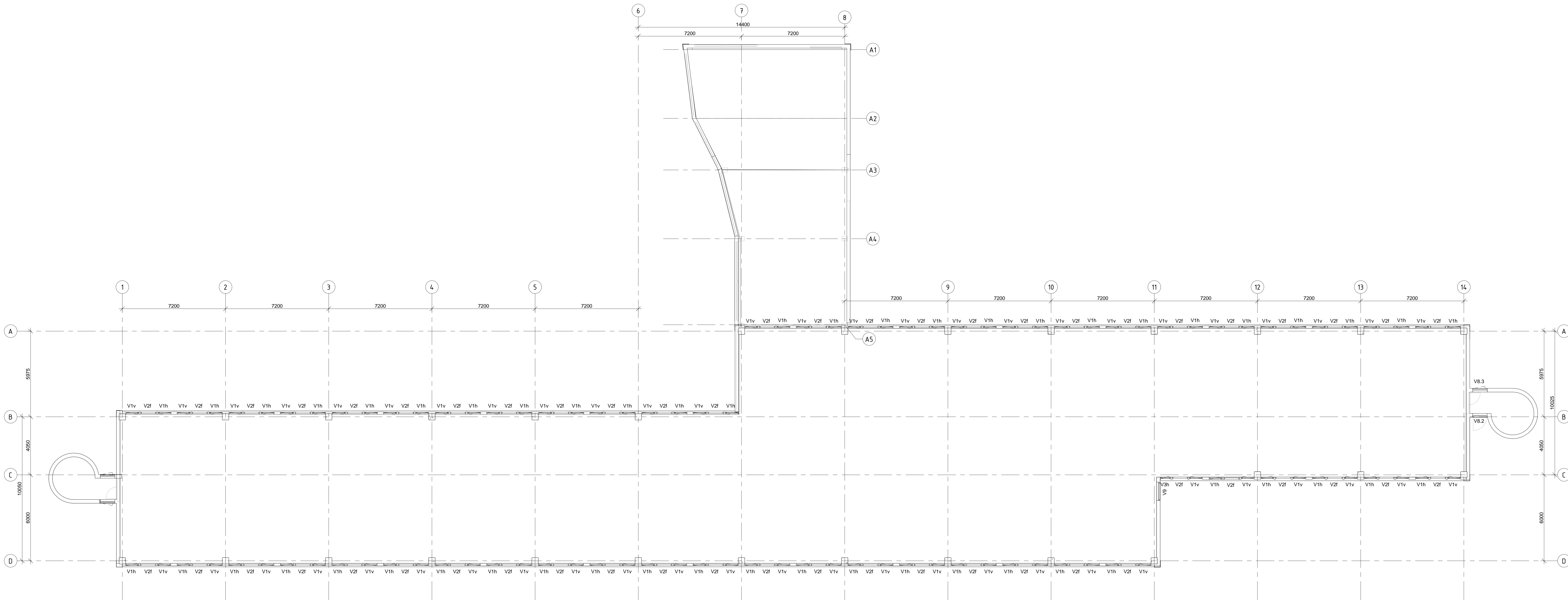
Plan 02 1 : 100
