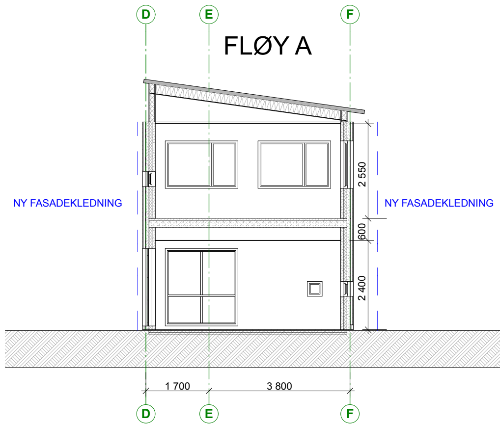
SNITT A
