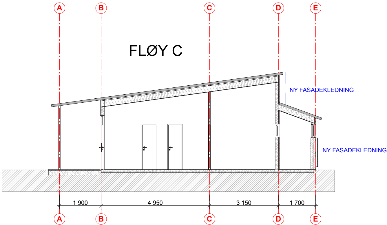
SNITT C
