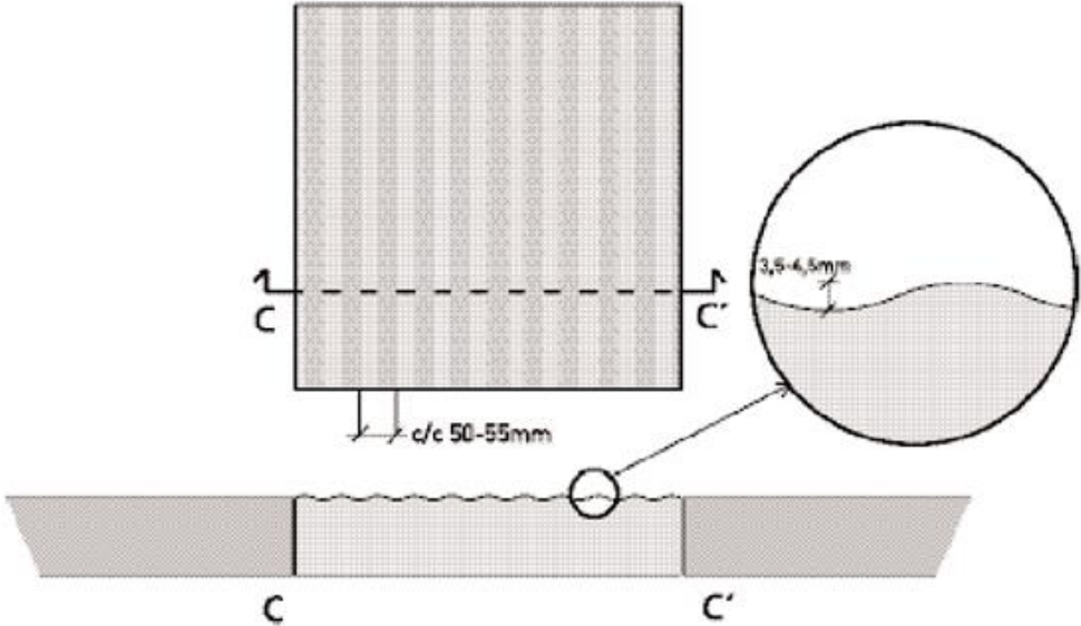
Figur 6: Retningsindikator utformet som sinushelle. Figuren viser høyde og c/c-avstand på ribbene.
