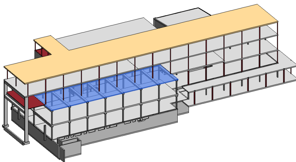
Figur 3-1: 3D-illustrasjon bæresystem
