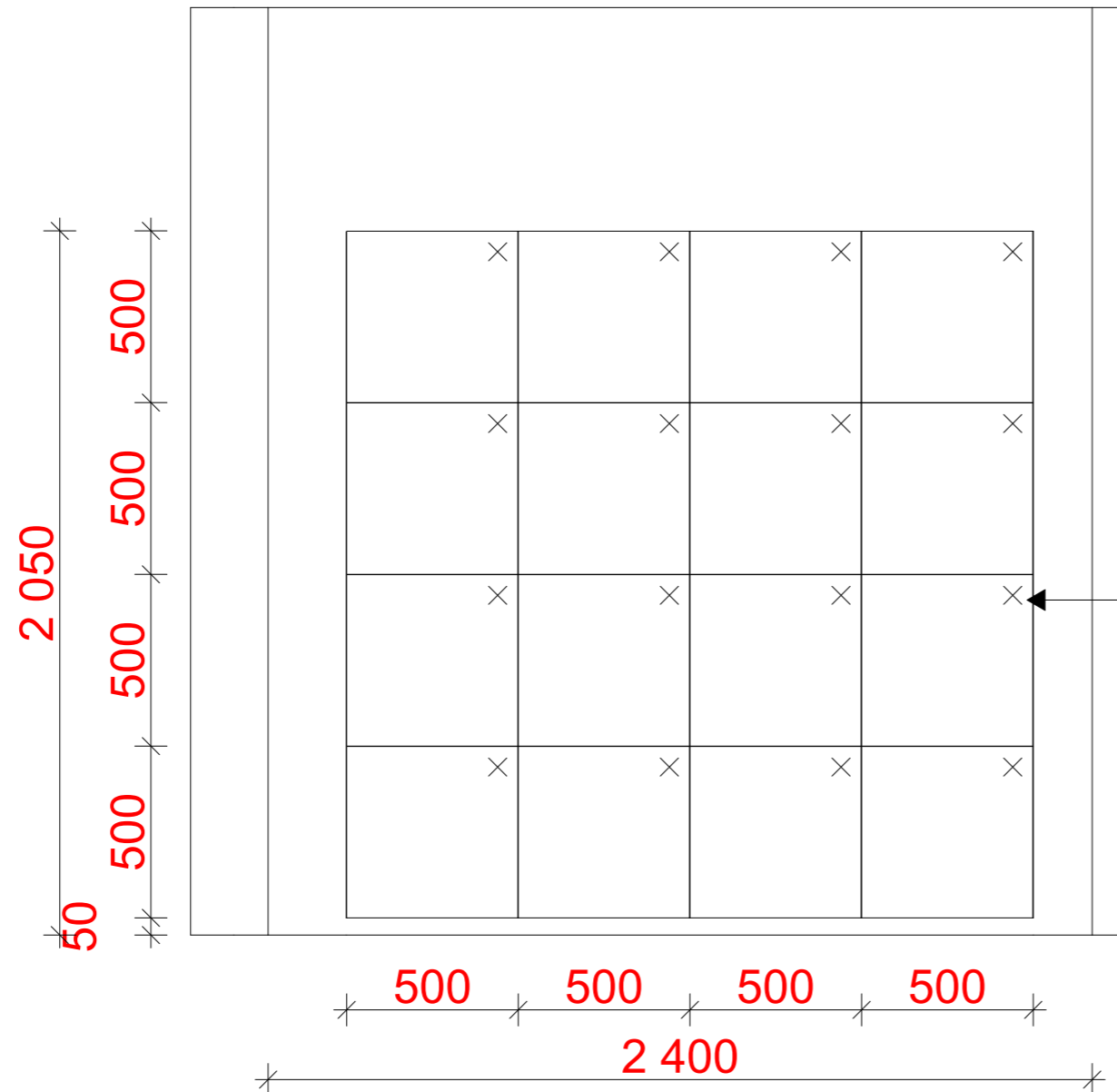
OPPRISS AA 1:20
