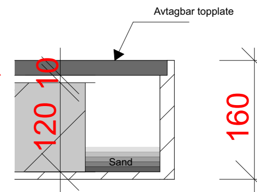
DETALJ A 1:5
