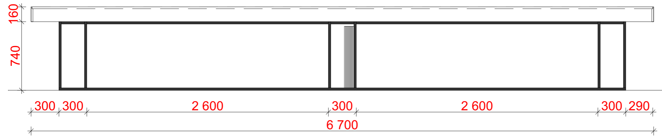
OPPRISS AA 1:25
