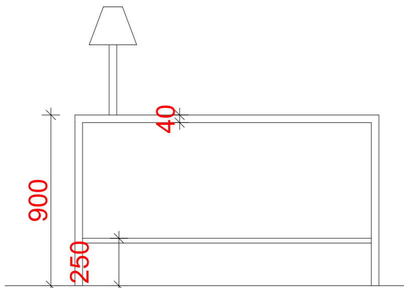
OPPRISS AA 1:20
