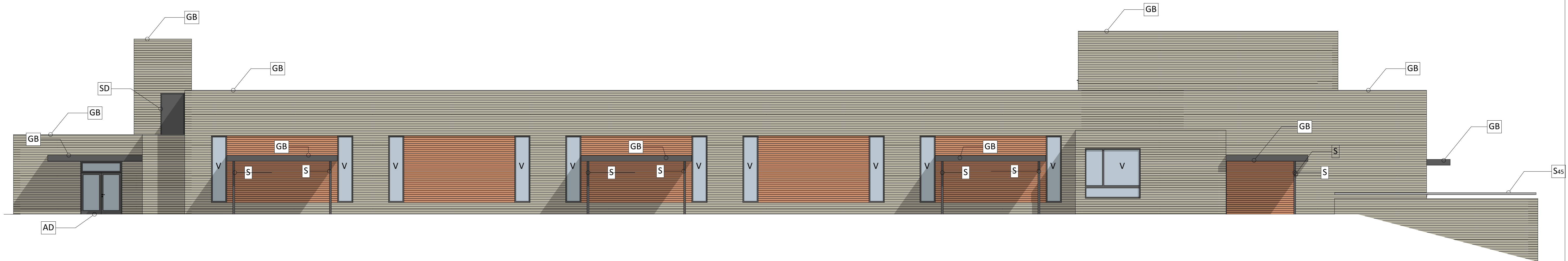
FASADE NORD
