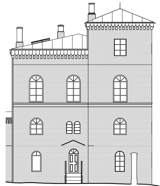
2 Fasade F-2 1 : 200
