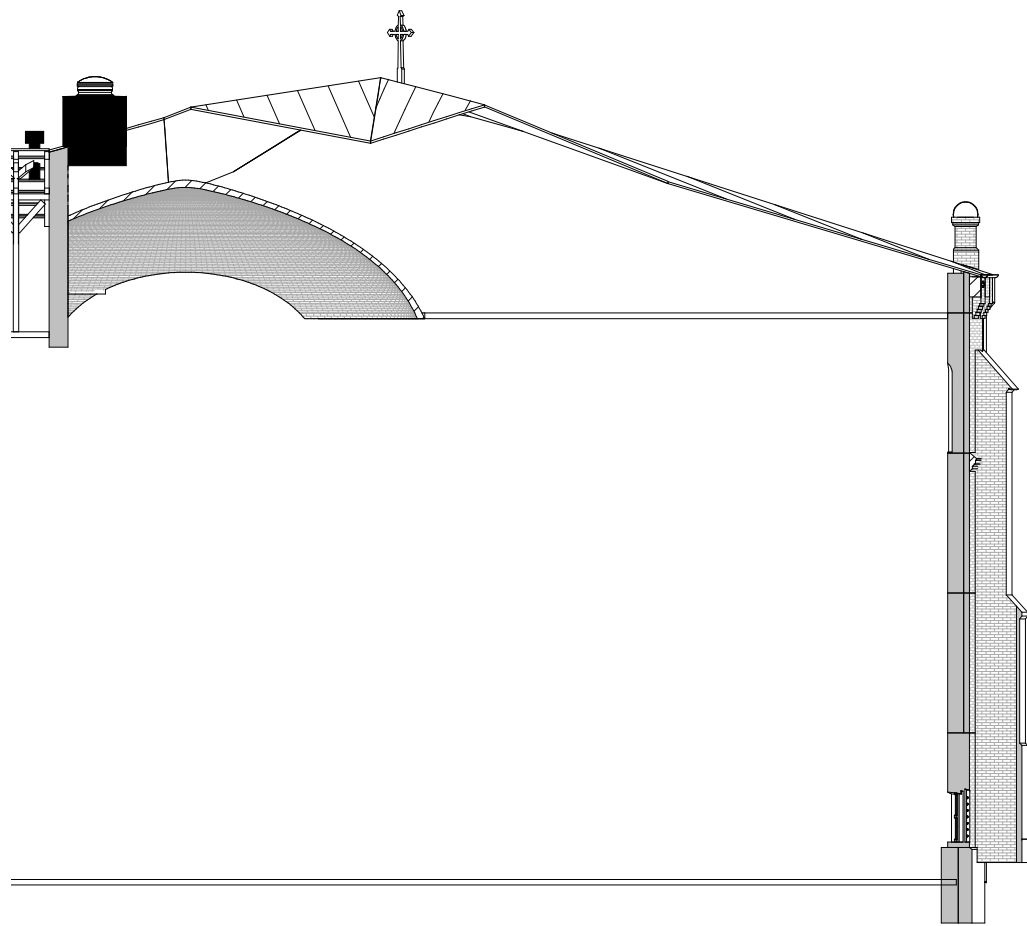
1 Snitt Midtbygget 1 : 200
