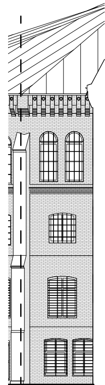
1 Fasade M-1 1 : 200
