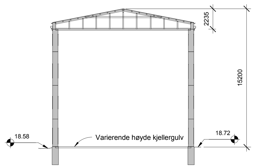
2 Tverrsnitt fløy D 1 : 200
