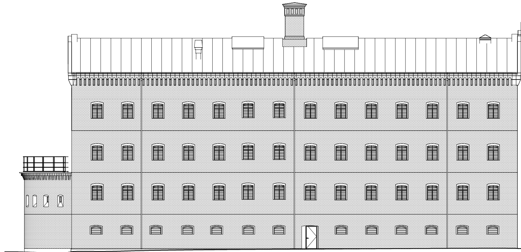
1 Fasade A-1 1 : 200
