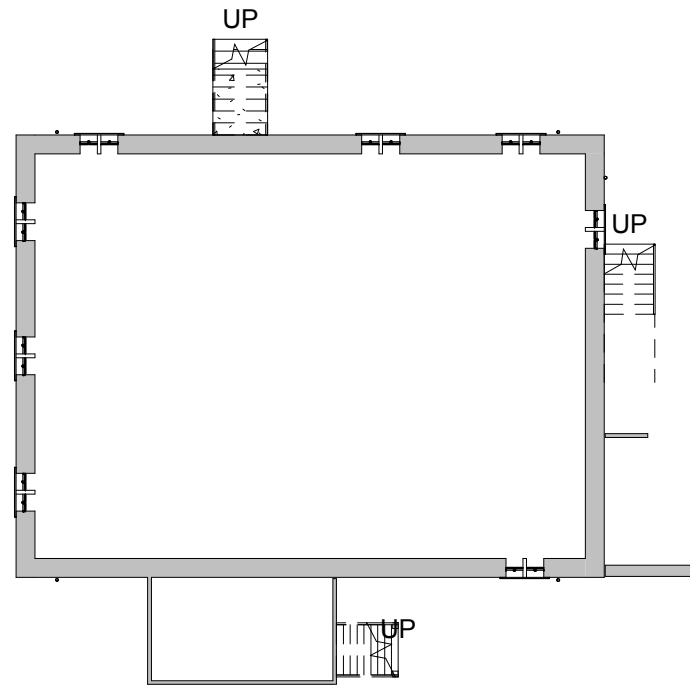
1 Plan UE bygg G 1 : 200
