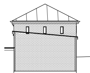
3 Fasade H-3 1 : 200
