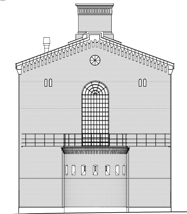
1 Fasade B-2 1 : 200
