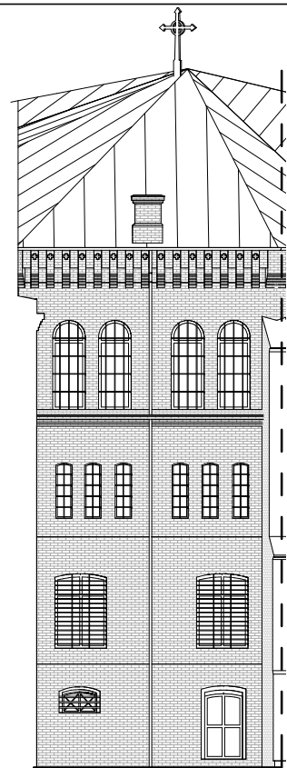
2 Fasade M-2 1 : 200
