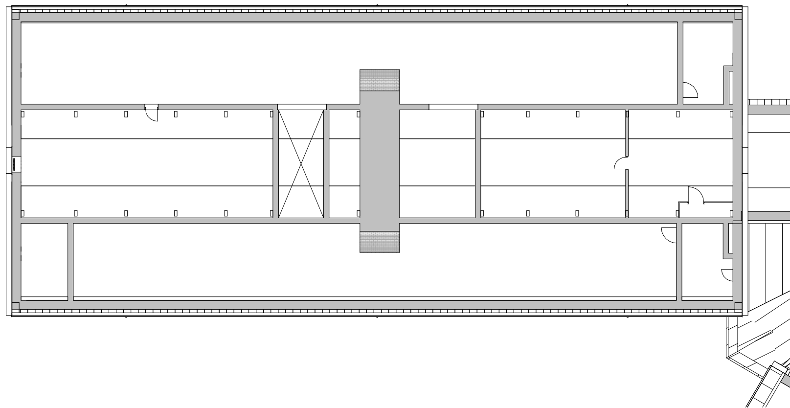
2 Plan 4 fløy C 1 : 200
