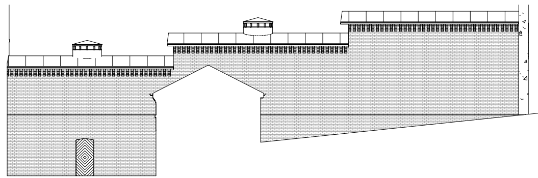
2 Fasade T-2 1 : 200
