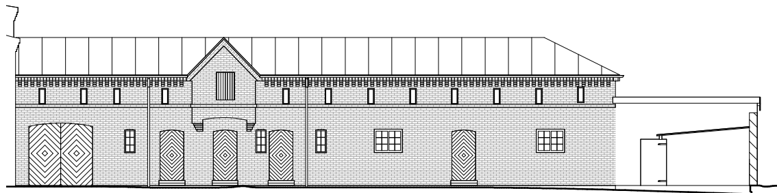
1 Fasade H-1 1 : 200
