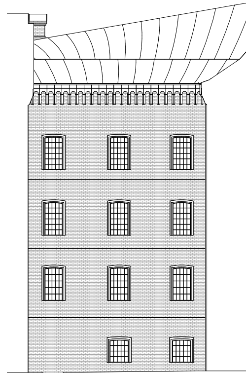
1 Fasade A-1 1 : 200
