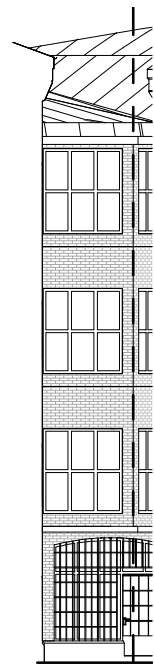
6 Fasade M-5b 1 : 200
