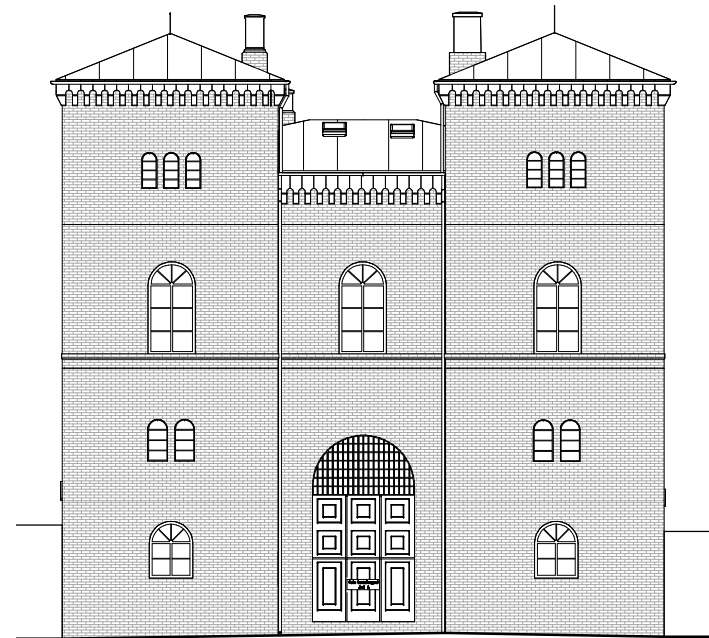
1 Fasade F-1 1 : 200
