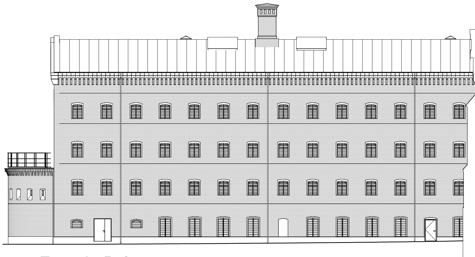
1 Fasade B-2 1 : 200
