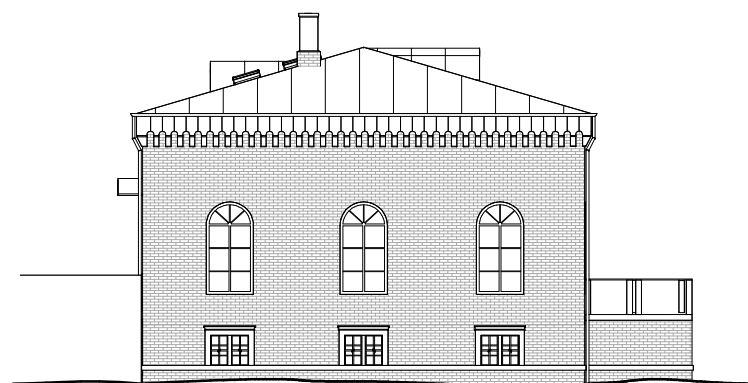
1 Fasade G-1 1 : 200
