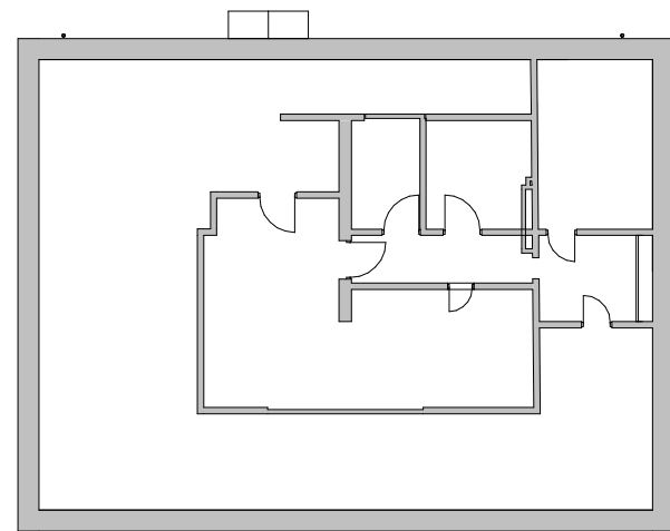
3 Plan 2 bygg G 1 : 200
