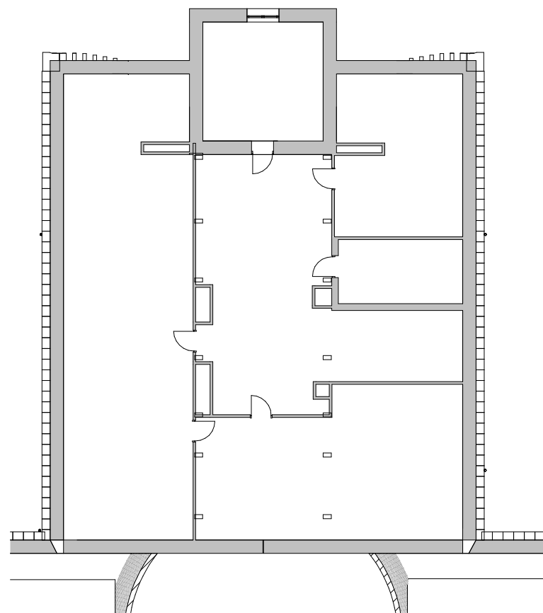
1 Plan 4 fløy E 1 : 200
