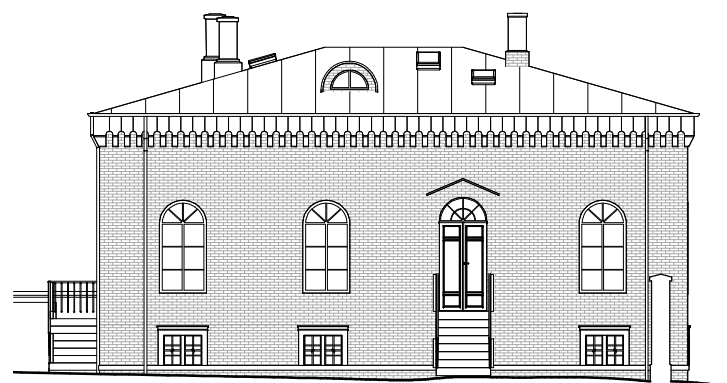
2 Fasade G-2 1 : 200
