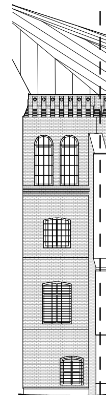
4 Fasade M-4 1 : 200
