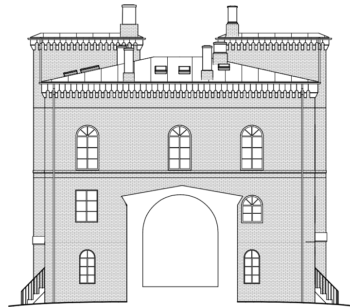
3 Fasade F-3 1 : 200
