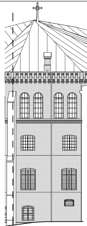
3 Fasade M-3 1 : 200
