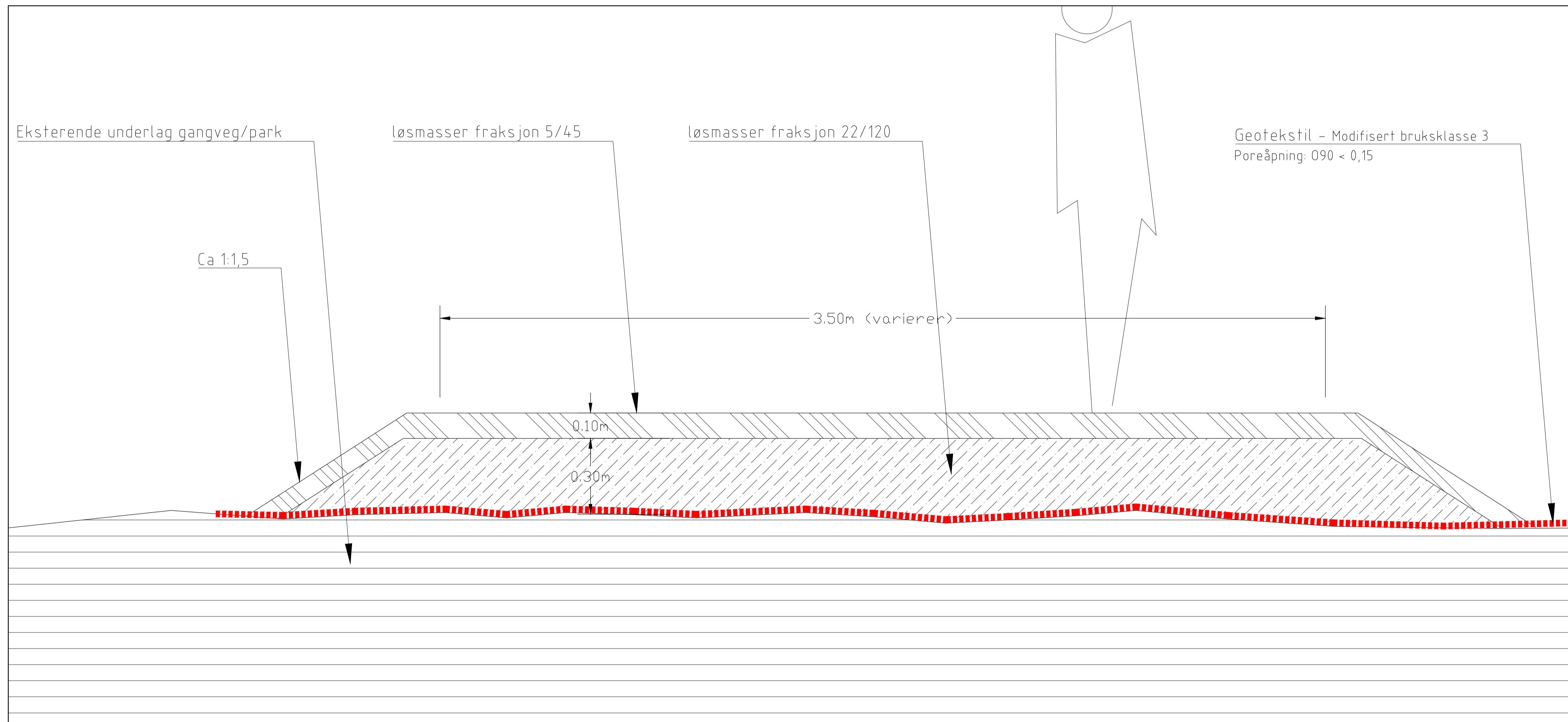
snitt midlertidig anleggsveg og riggområde 1:10
