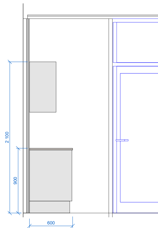
Sideoppriss 1 : 25
