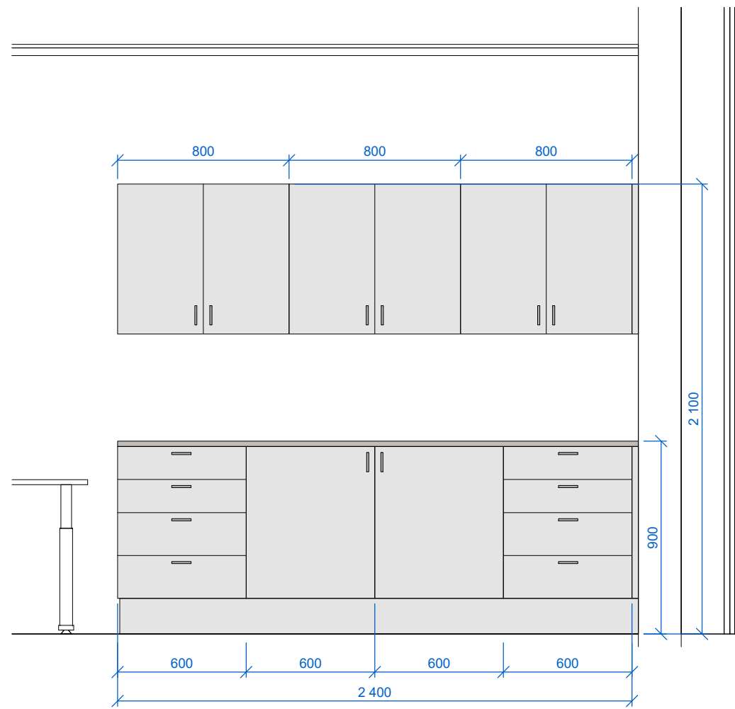
Oppriss 1 : 25
