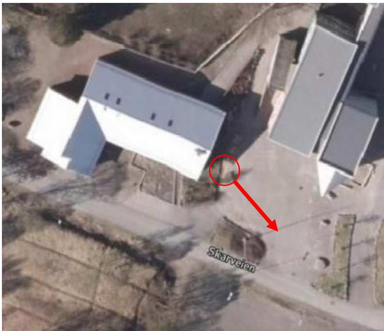
Kum 123 detaljfoto Eksisterende stakekum 123 SP 110 og OV 110
