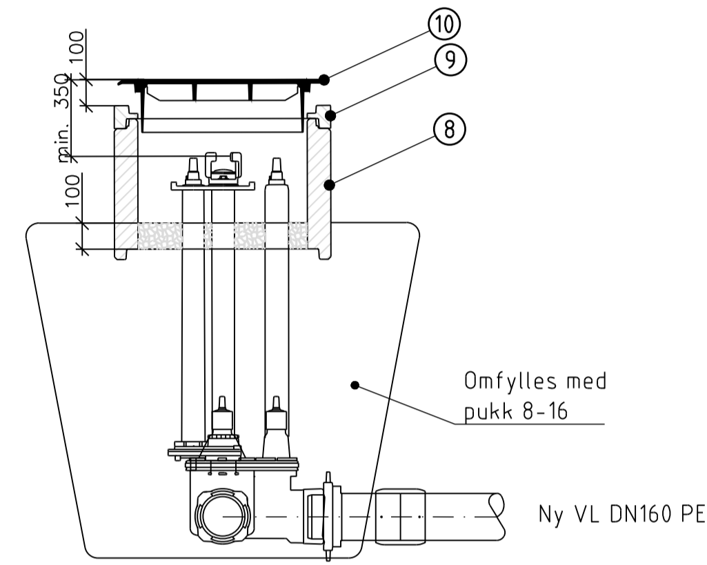
Snitt VK2
