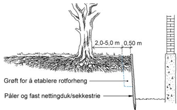
Fig. 561 Eksempel på rotforheng ved terrenginngrep
