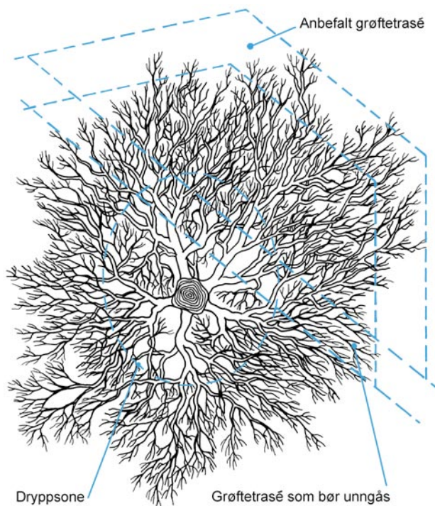
Fig. 26 Planlegg slik at grøfter og rør ikke føres gjennom trærnes rotsoner.
