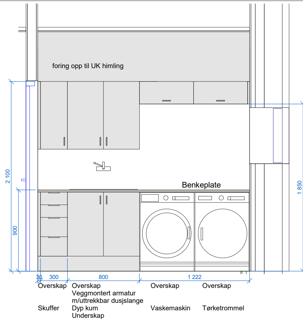
_Oppriss vask/tørk 1 : 25
