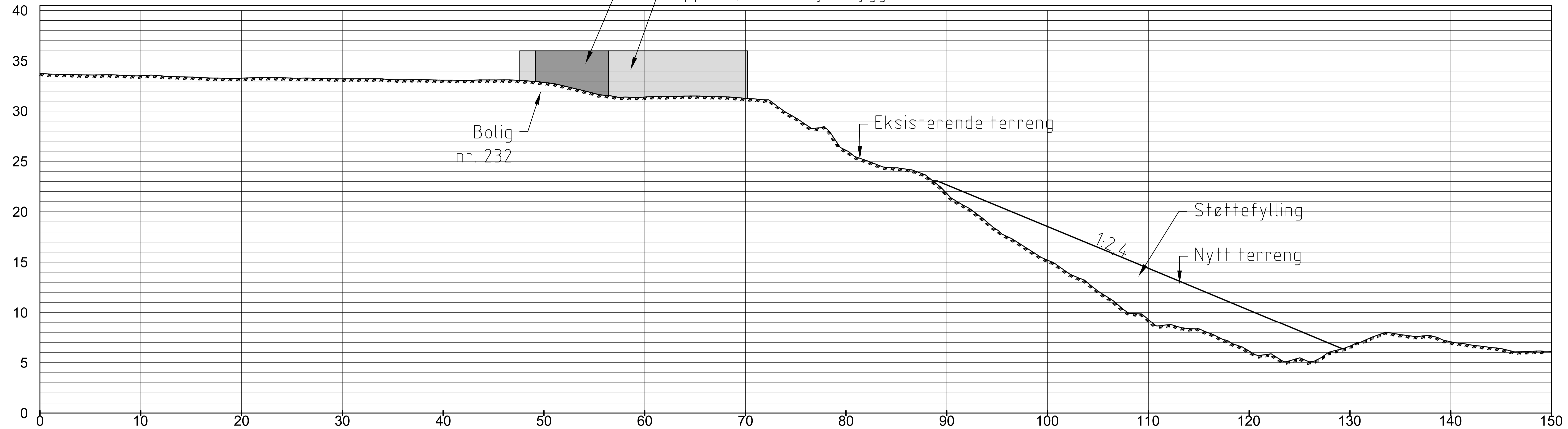
Snitt 4 M=1:500 A3
