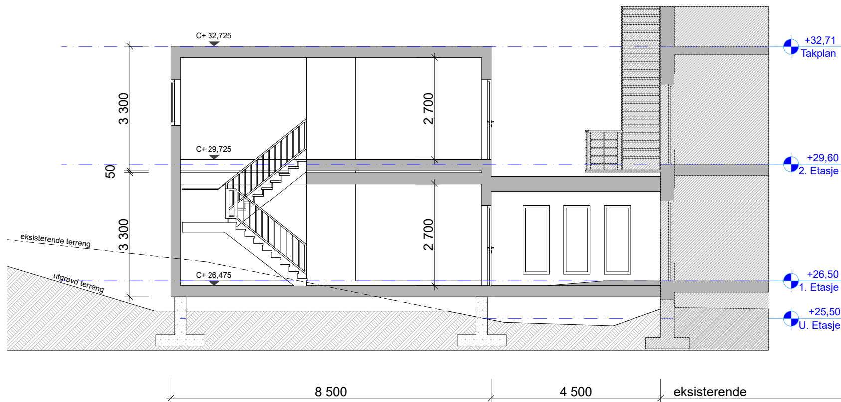
1:100 Snitt A
