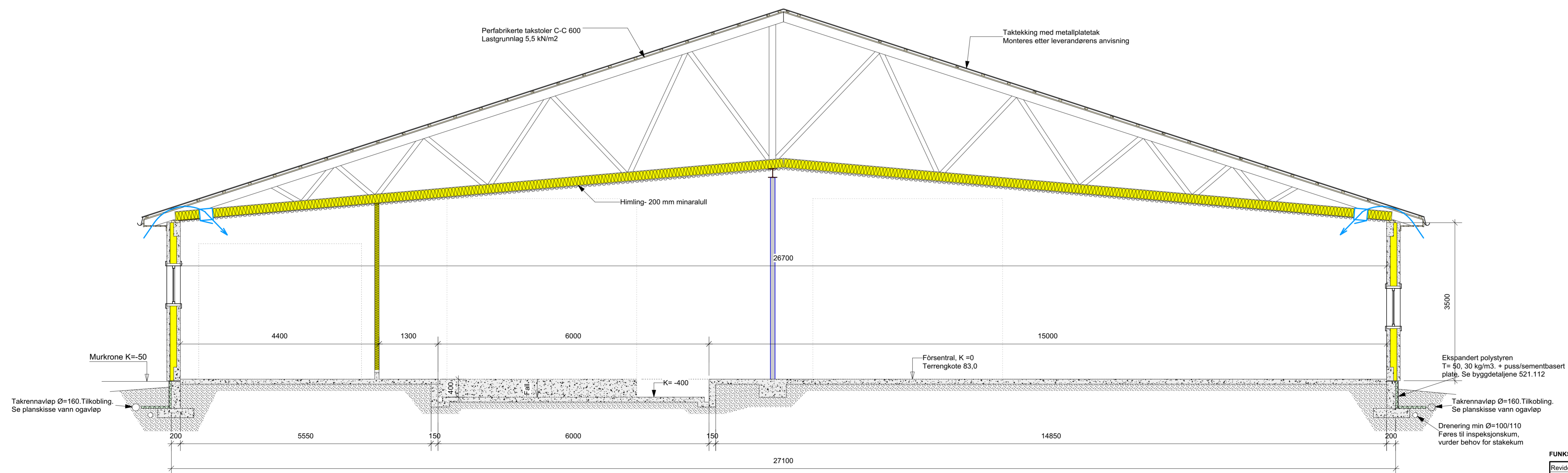
SNITT D-D. 1:50
