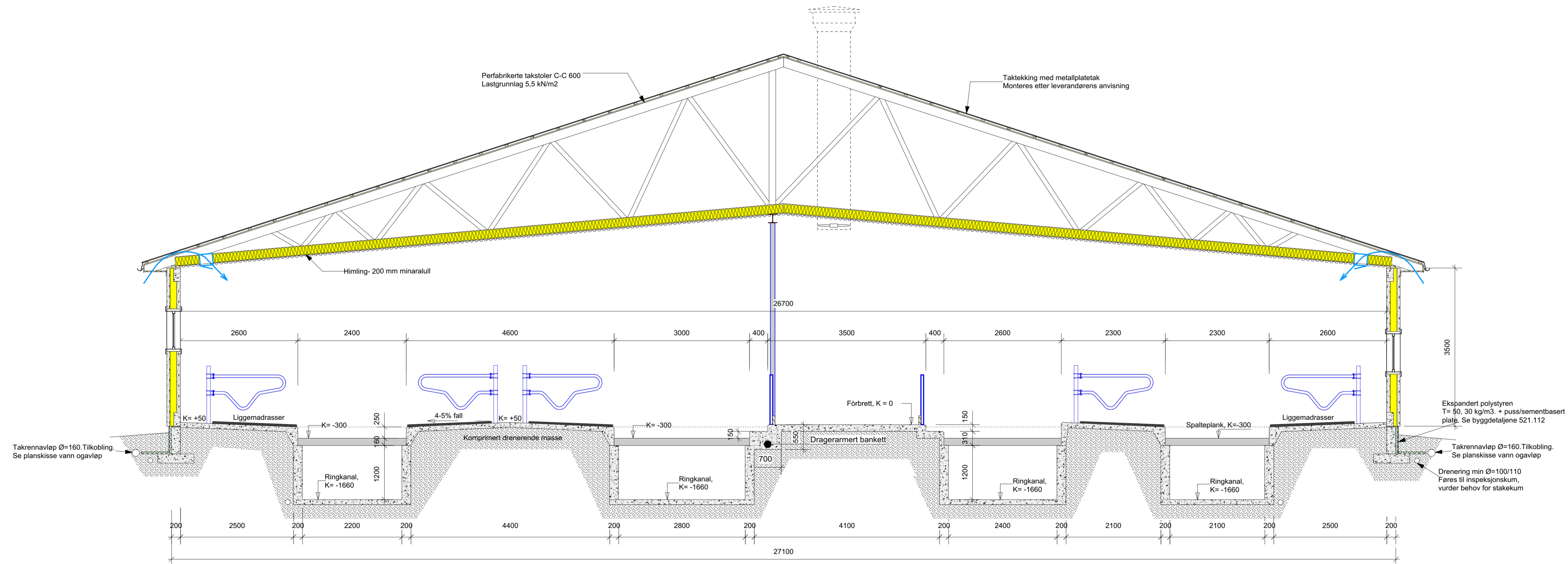
SNITT C-C. 1:50
