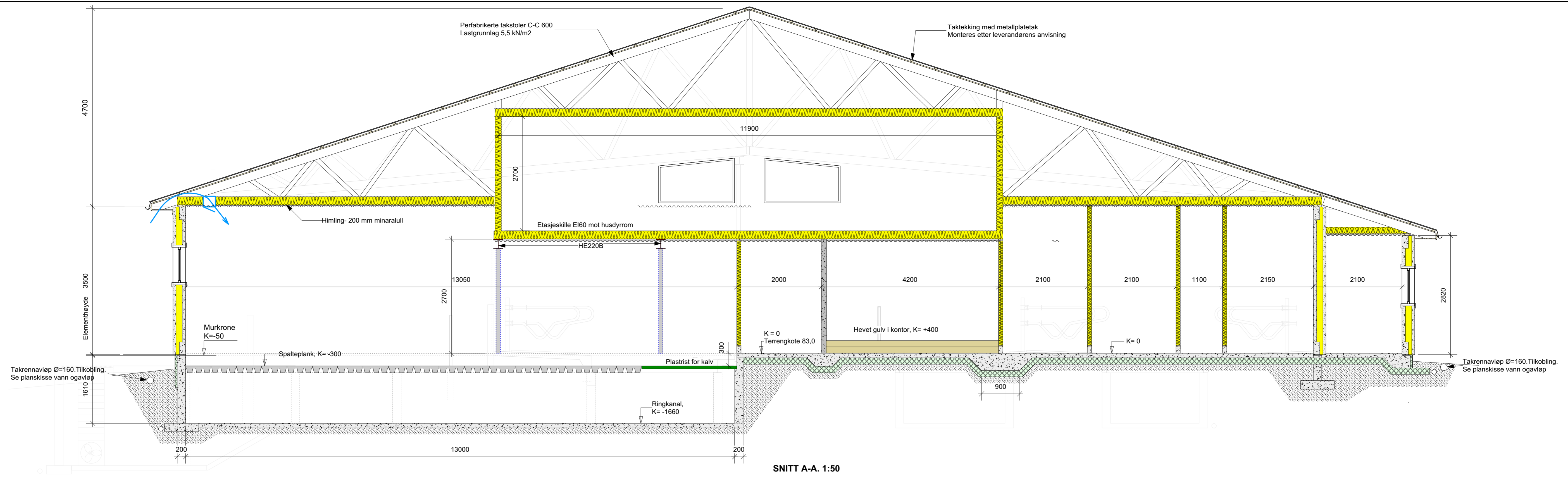
SNITT A-A. 1:50
