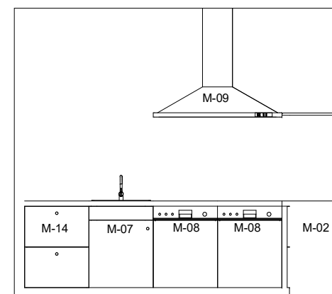
101-3 Steril 1:50
