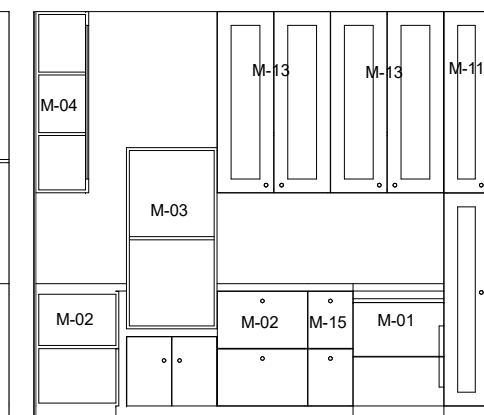
101-4 Steril 1:50
