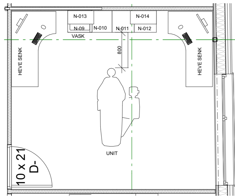
Plan 1:50
