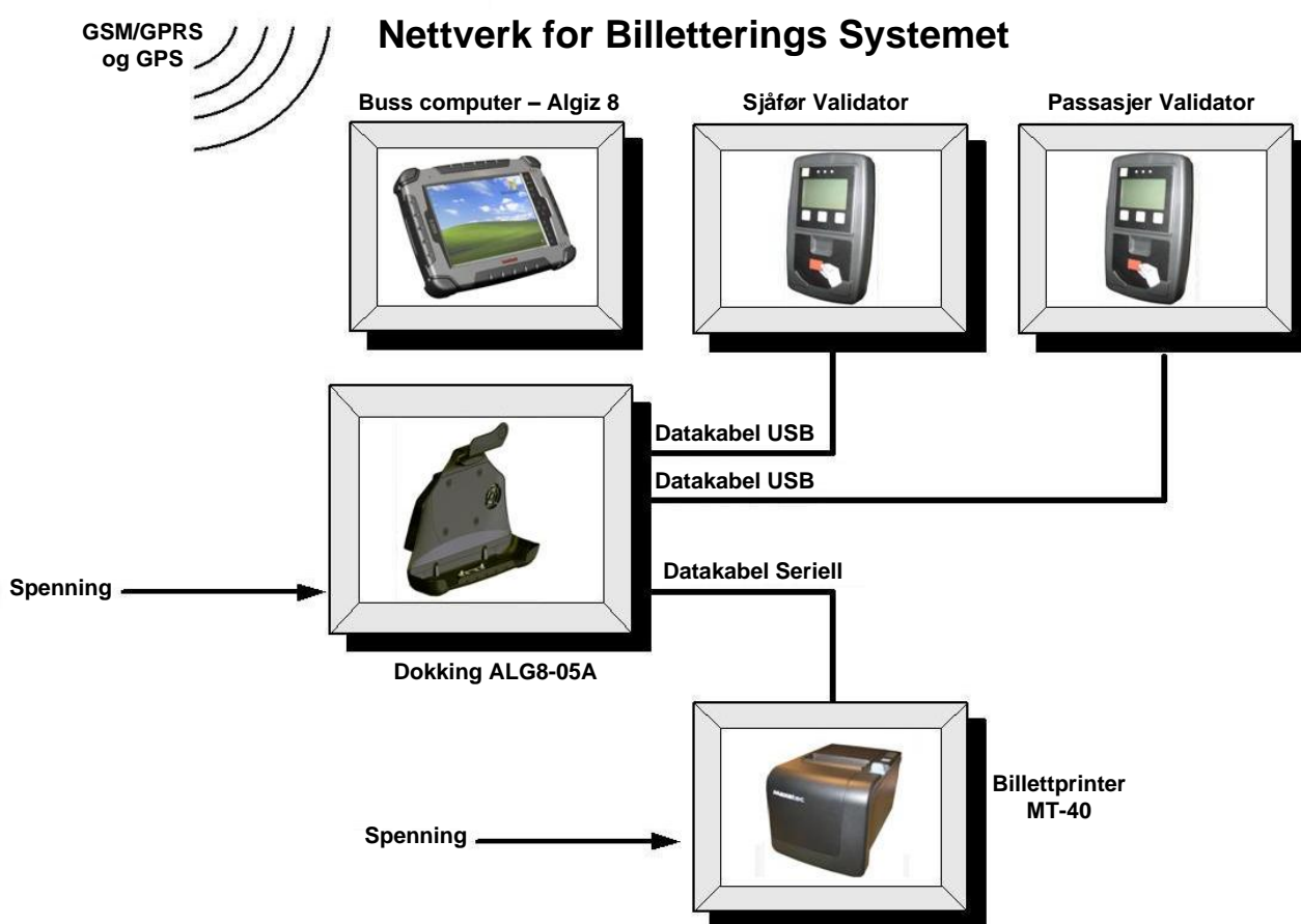
Figur 2 - Nettverk billetteringssystem
