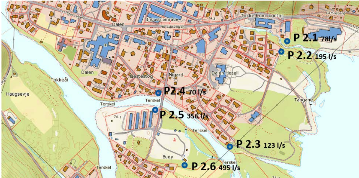
Fig 3.4.4.1 - Oversikt pumpeanlegg (Førebels pumpekapasitet)
