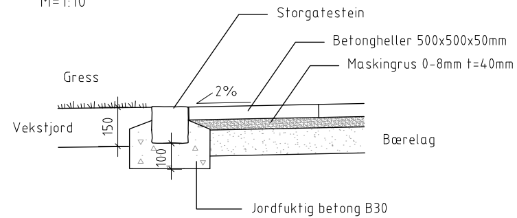
Snitt uteplasser betongheller M=1:10
