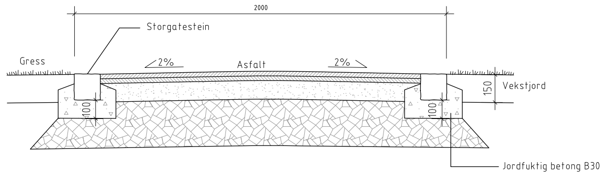
Snitt gangstier M=1:10
