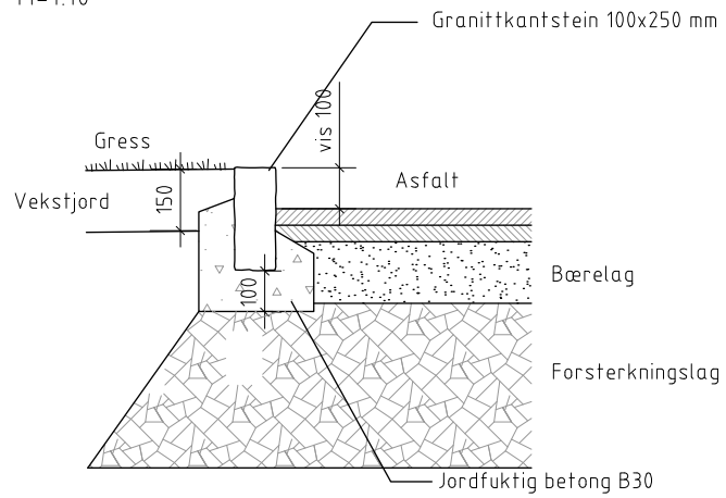
Snitt parkering M=1:10
