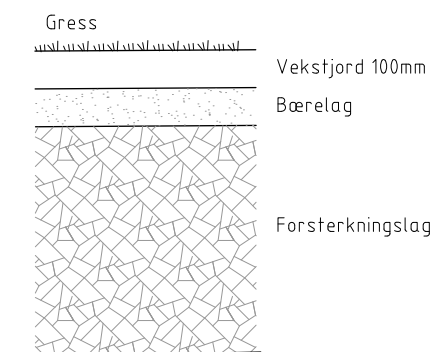
Snitt gress kjøsterkt M=1:10
