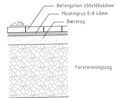
Snitt betongstein kjøsterkt M=1:10
