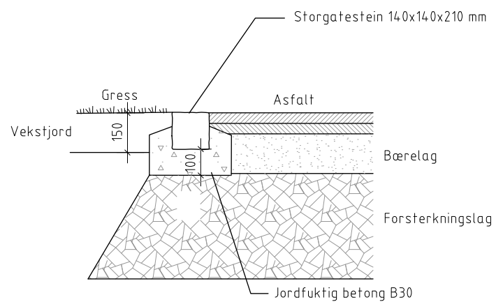
Snitt parkering mot bed M=1:10
