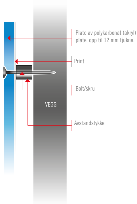
MONTERINGSPRINSIPP
