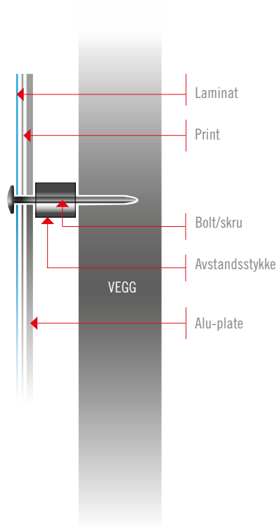
MONTERINGSPRINSIPP
