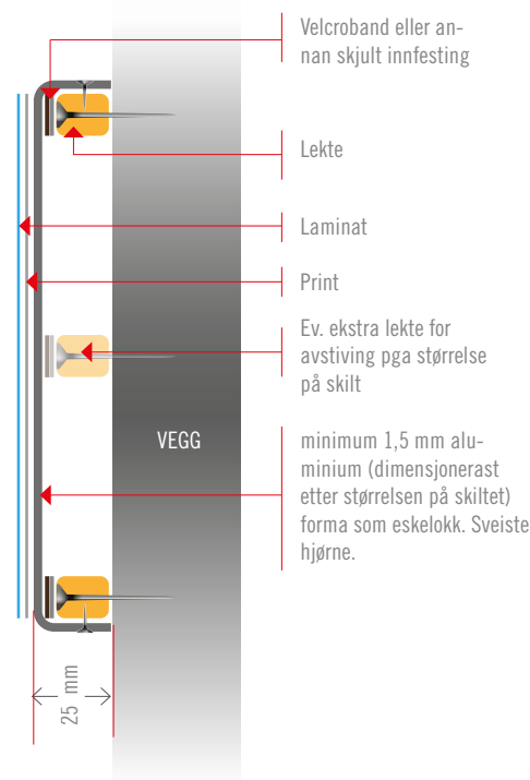
MONTERINGSPRINSIPP
