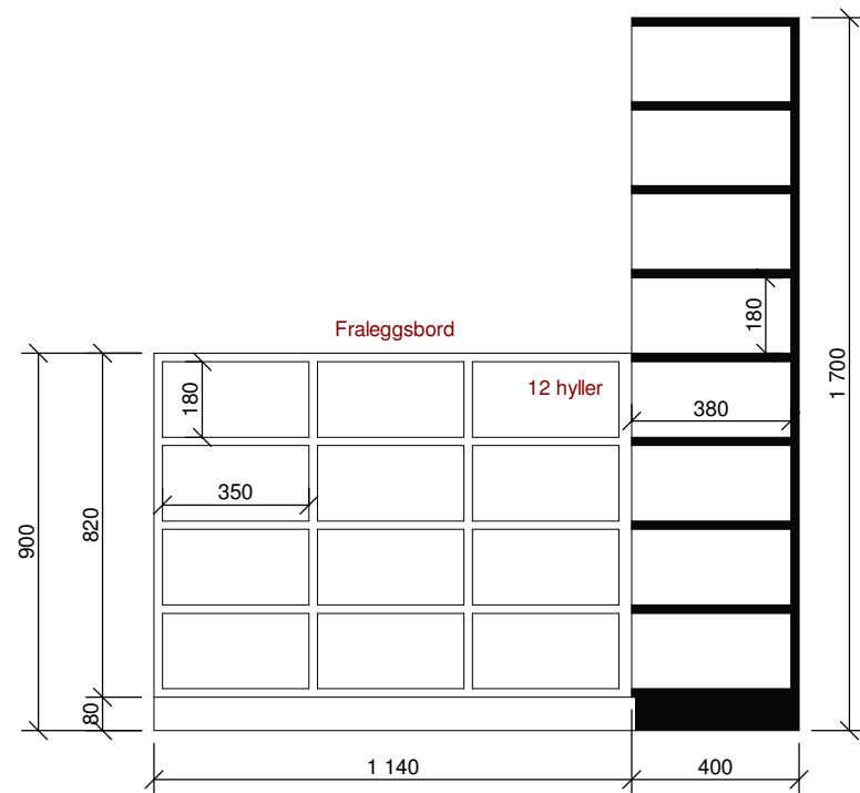
Snitt/ oppriss A
