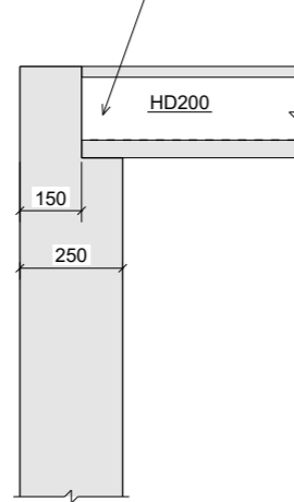
E - E 1:10
