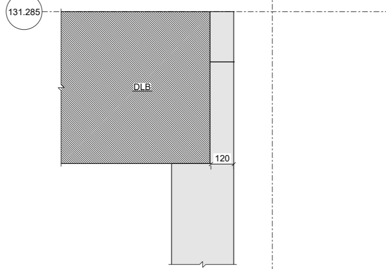
D - D 1:10
