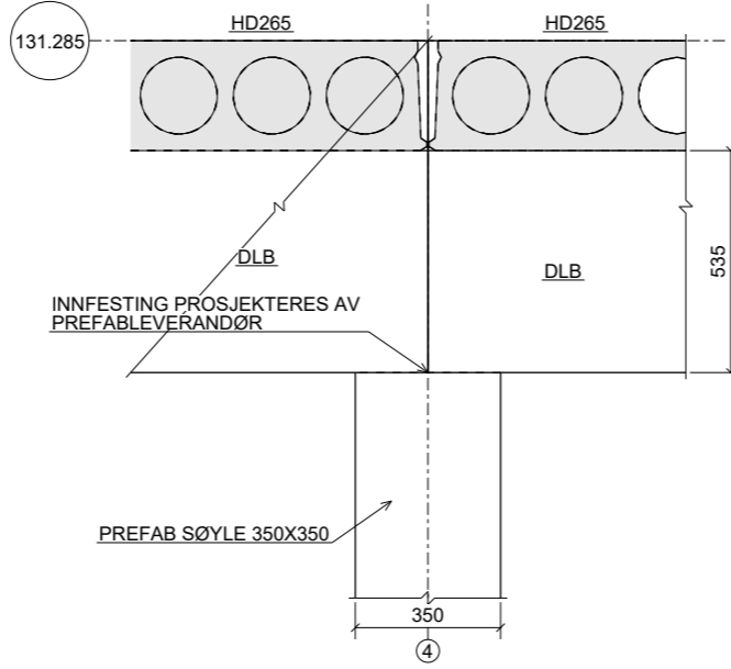
B - B 1:10
