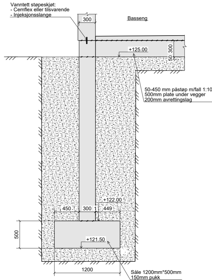
A - A 1:20
