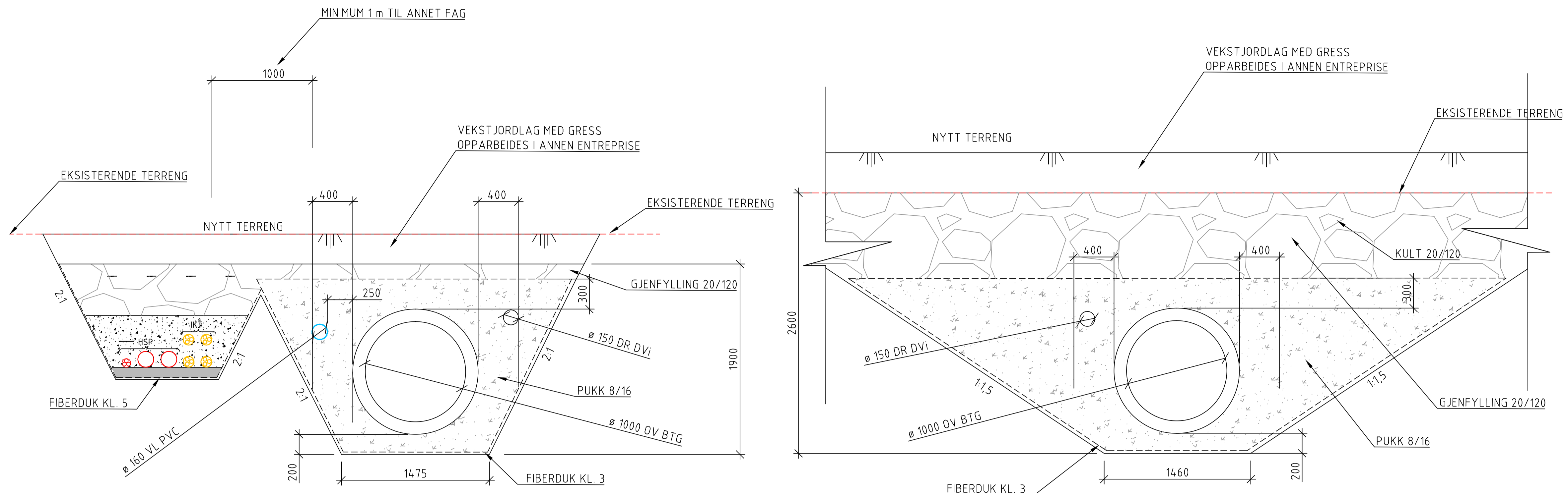
GRØFTESNITT ØV-KULVERT NORD PROFIL 50
