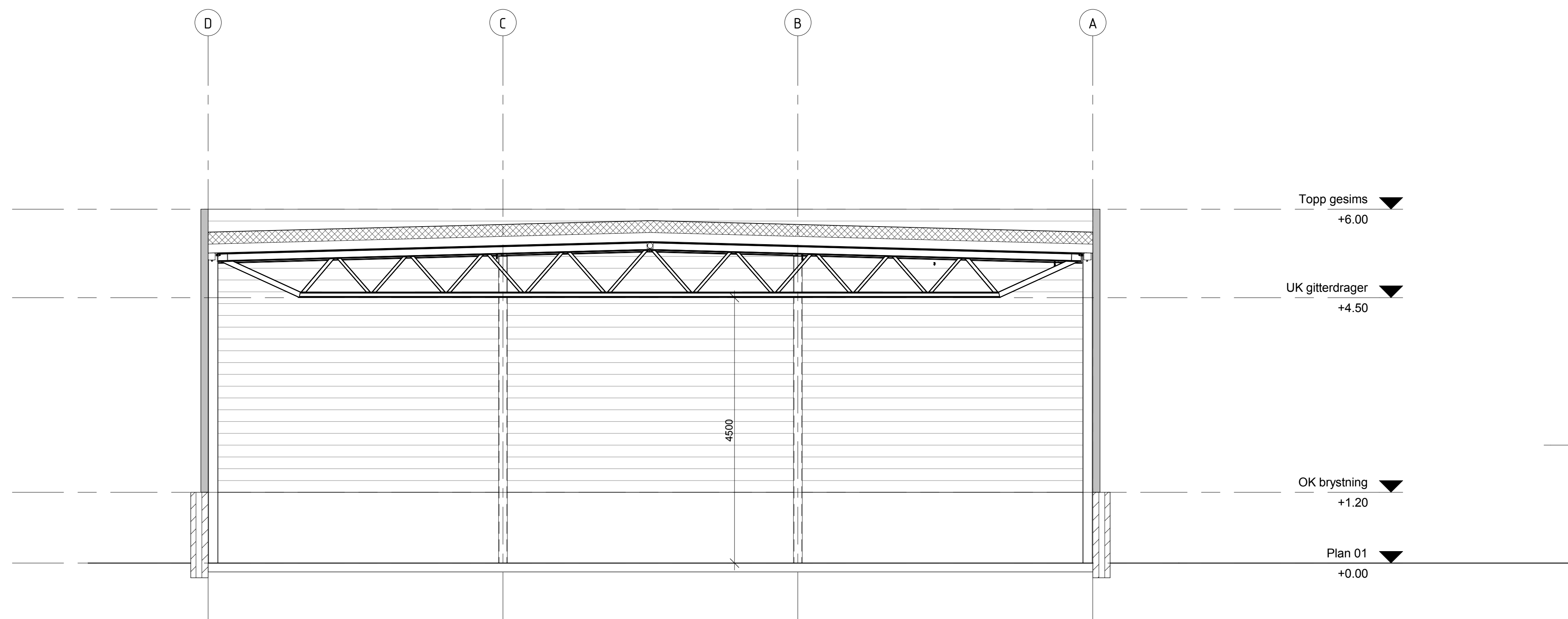
Snitt A-A 1 : 50
