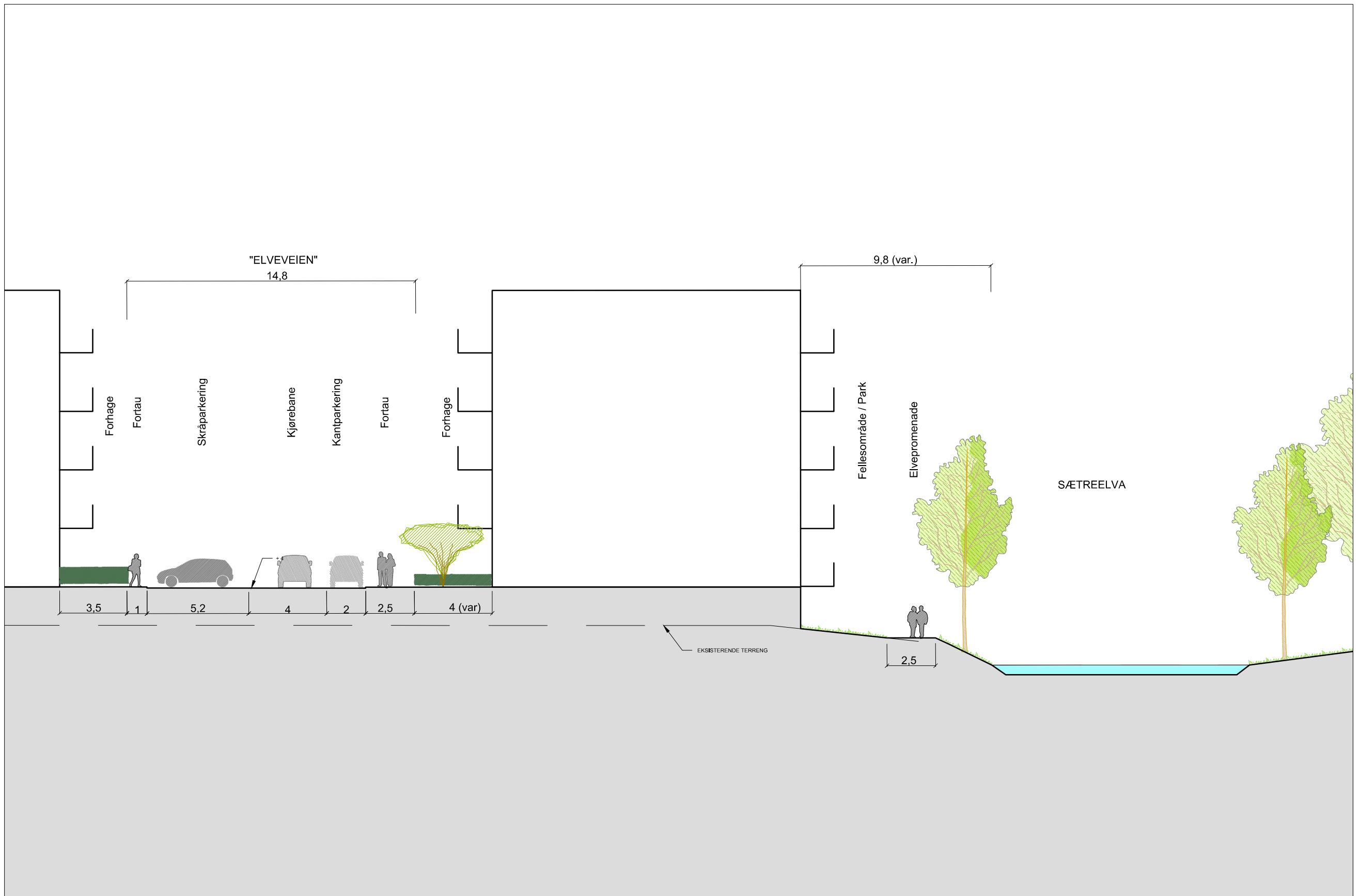
SNITT C - C' 1:200
