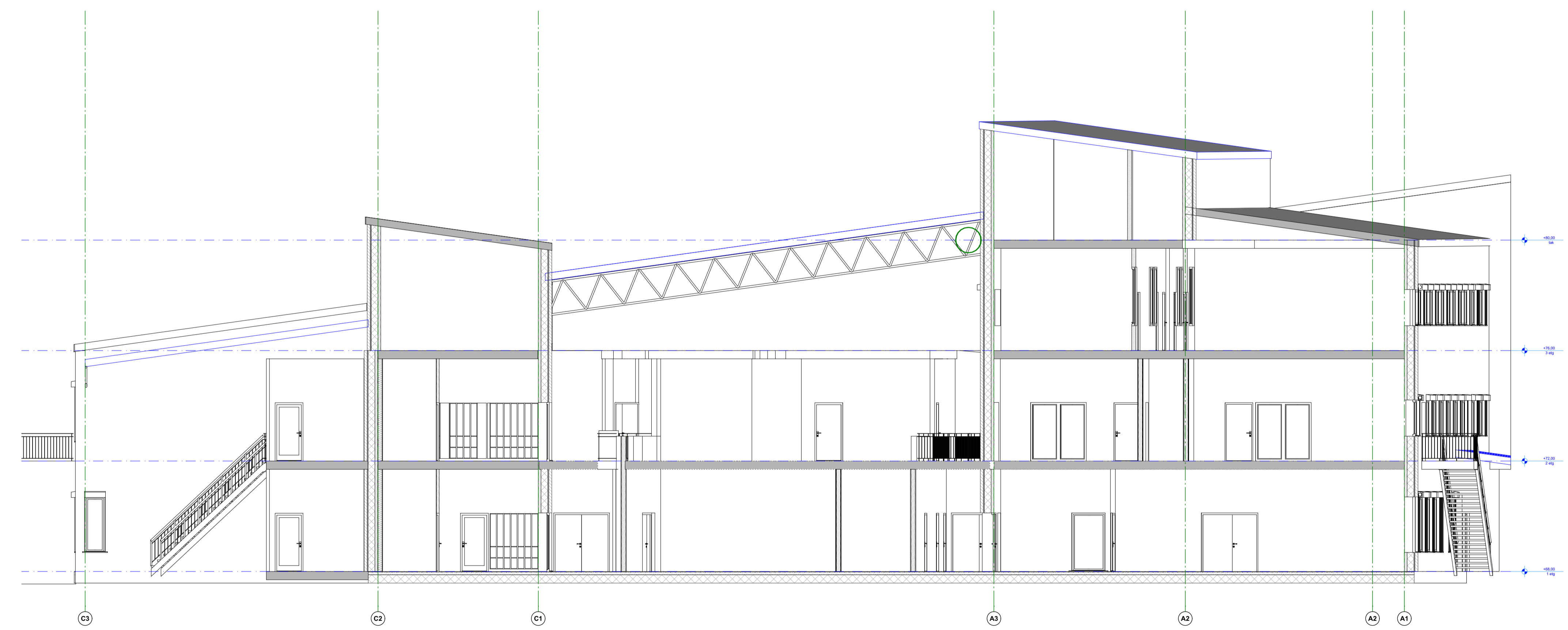
Tversnitt
