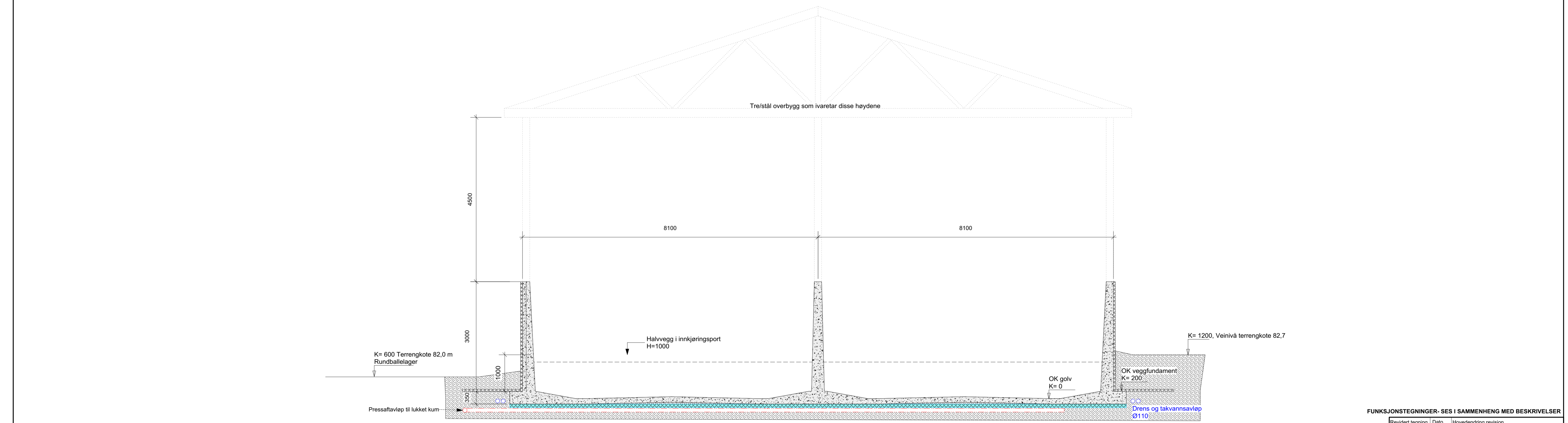
SNITT A-A, MALESTOKK 1:50
