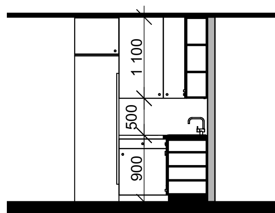
SNITT/ OPPRISS
