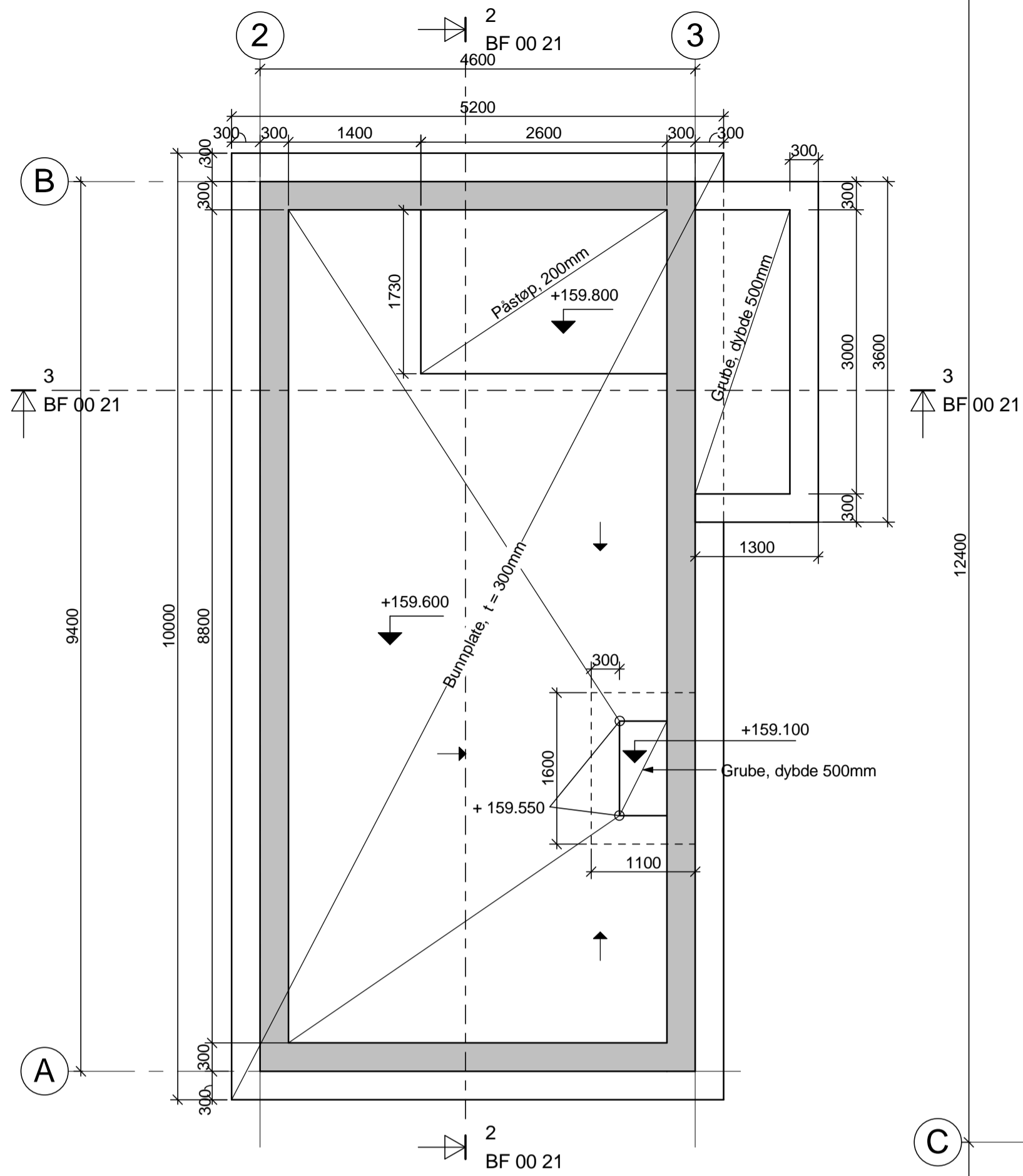
Fundamentplan - Kjeller 1 : 50
