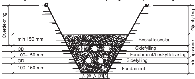
Figur 8. Grøfttverrsnitt pukk.
