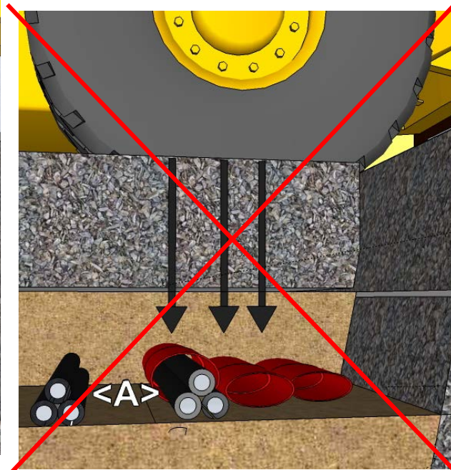
Figur 7 - RT9196 - Feil avstand ved legging av flere rør på ett nivå
