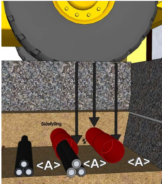
Figur 6 - RT9195 - Riktig avstand ved legging av flere rør på ett nivå
