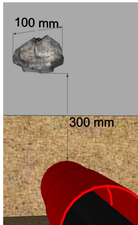
Figur 5 - RT9194 - Minste avstand fra stein til rør må være 3 ganger størrelsen av steinen
