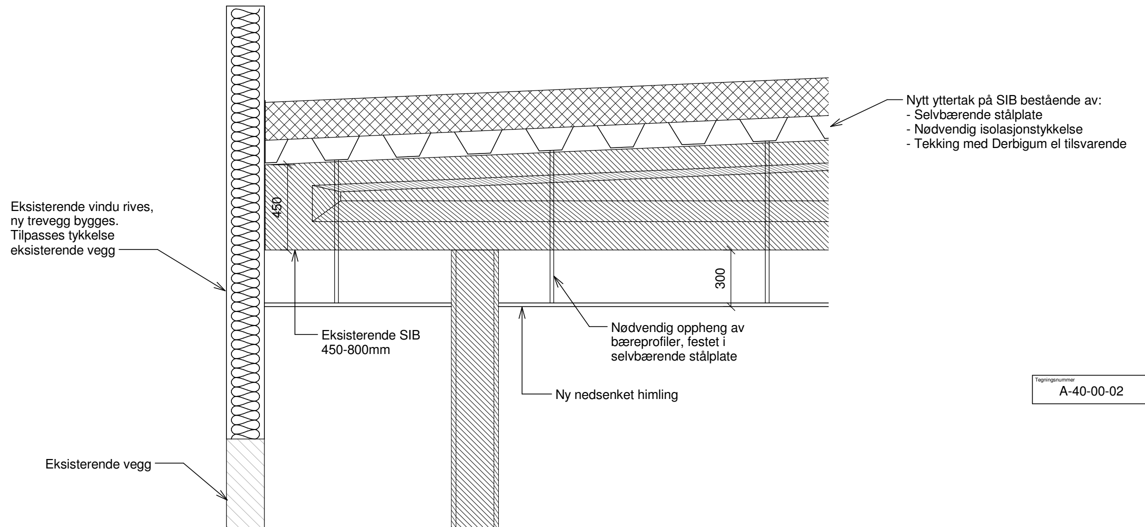
SNITT A 1 : 20
