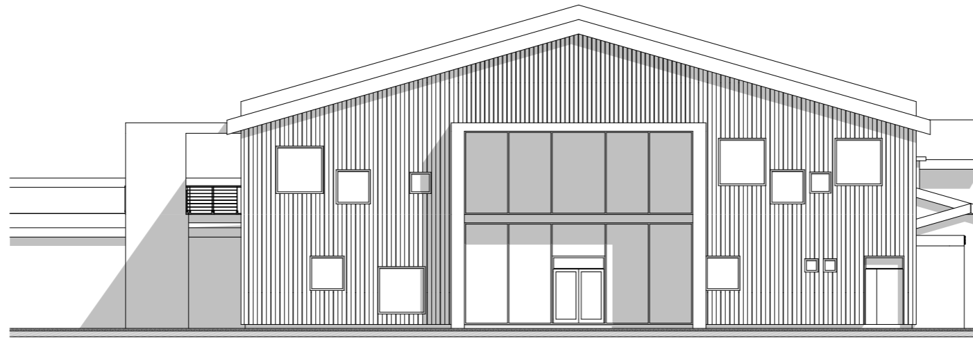
1:200 Fasade Sør-Vest
