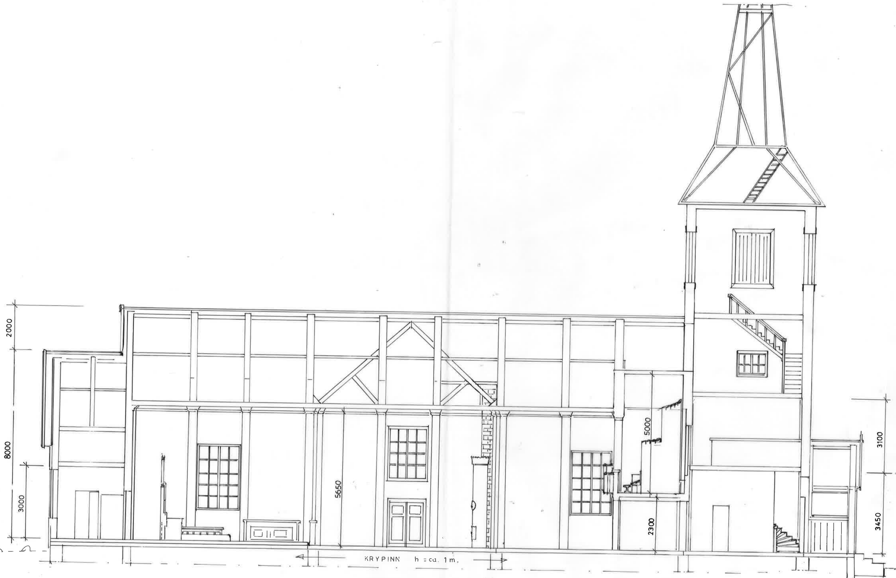
LENGDESNITT. ( I - I ).
