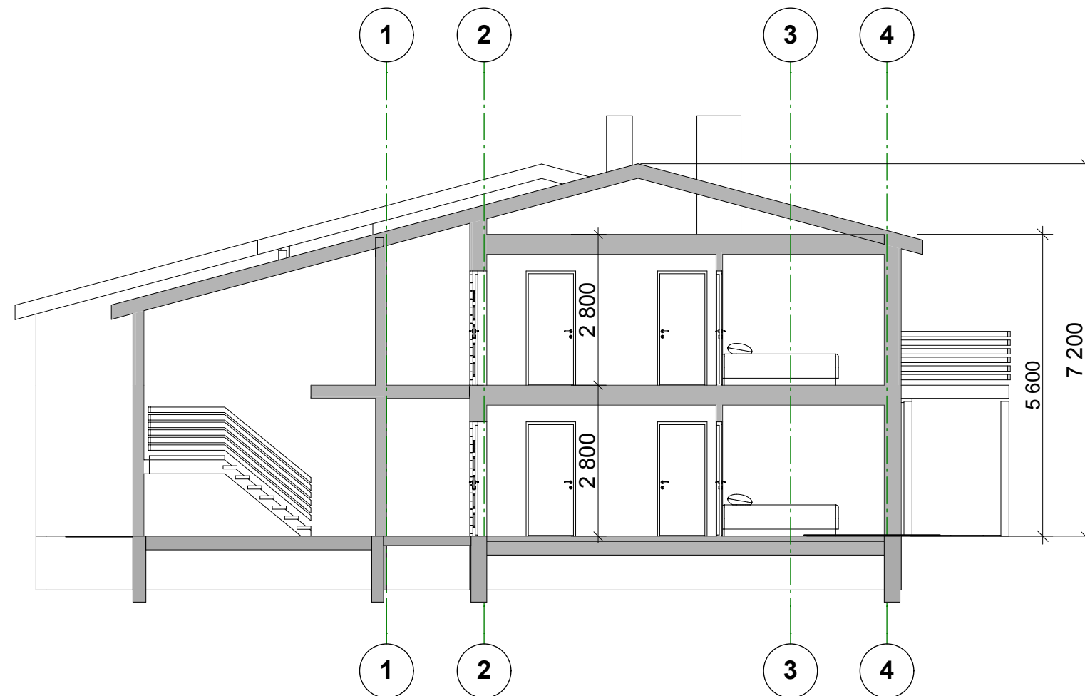
Snitt 1
