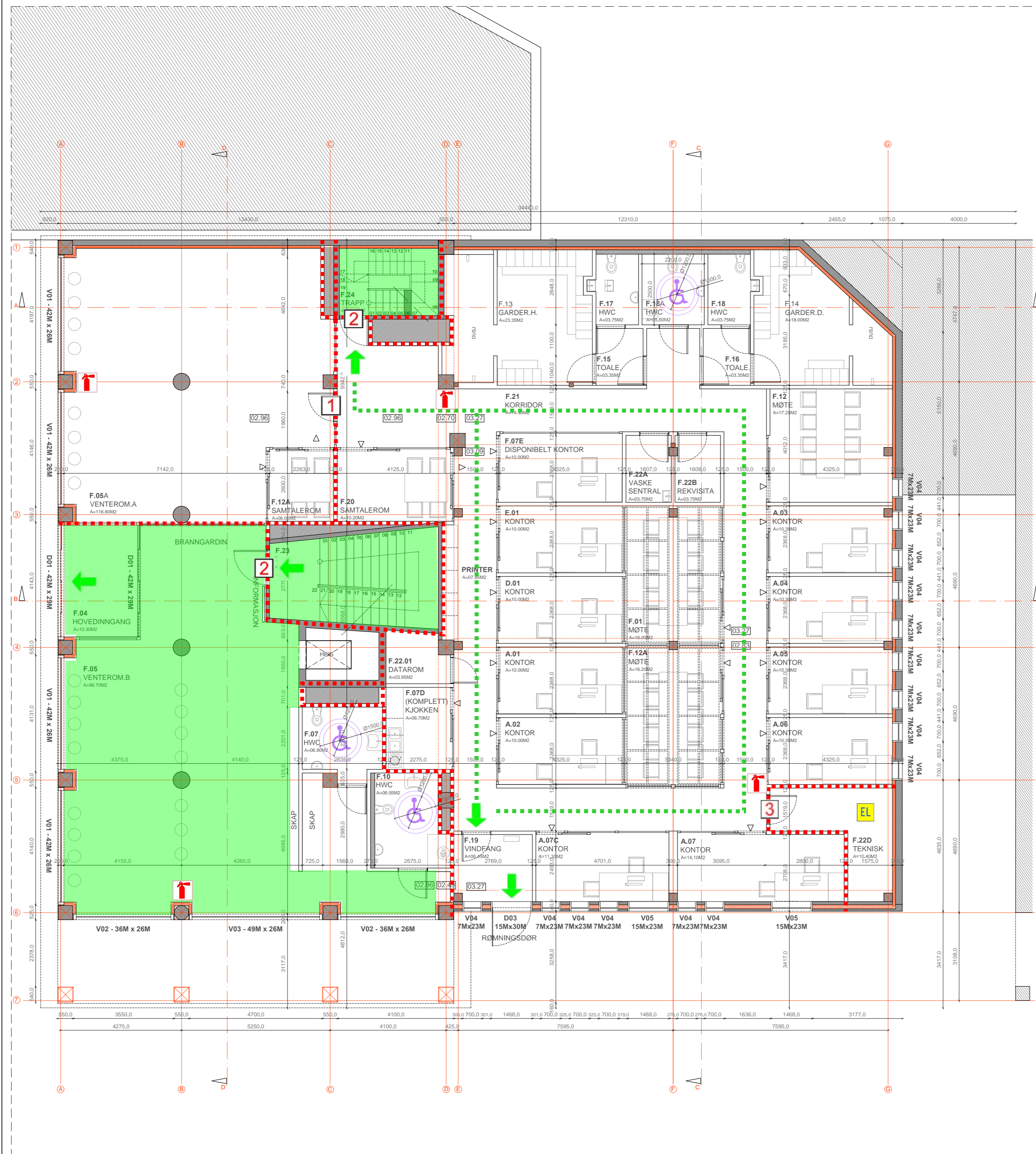
PLAN 1. ETASJE - (UNDER ARBEID: DIMENSJONER KREVJE BEKREFTELSE) PLAN M=1:100
