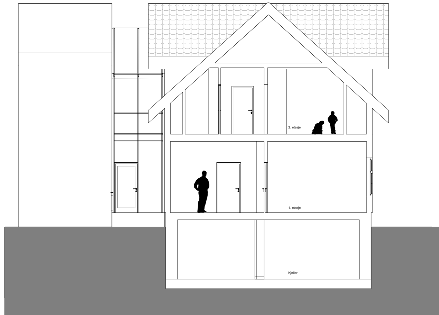
1:100 Snitt A
