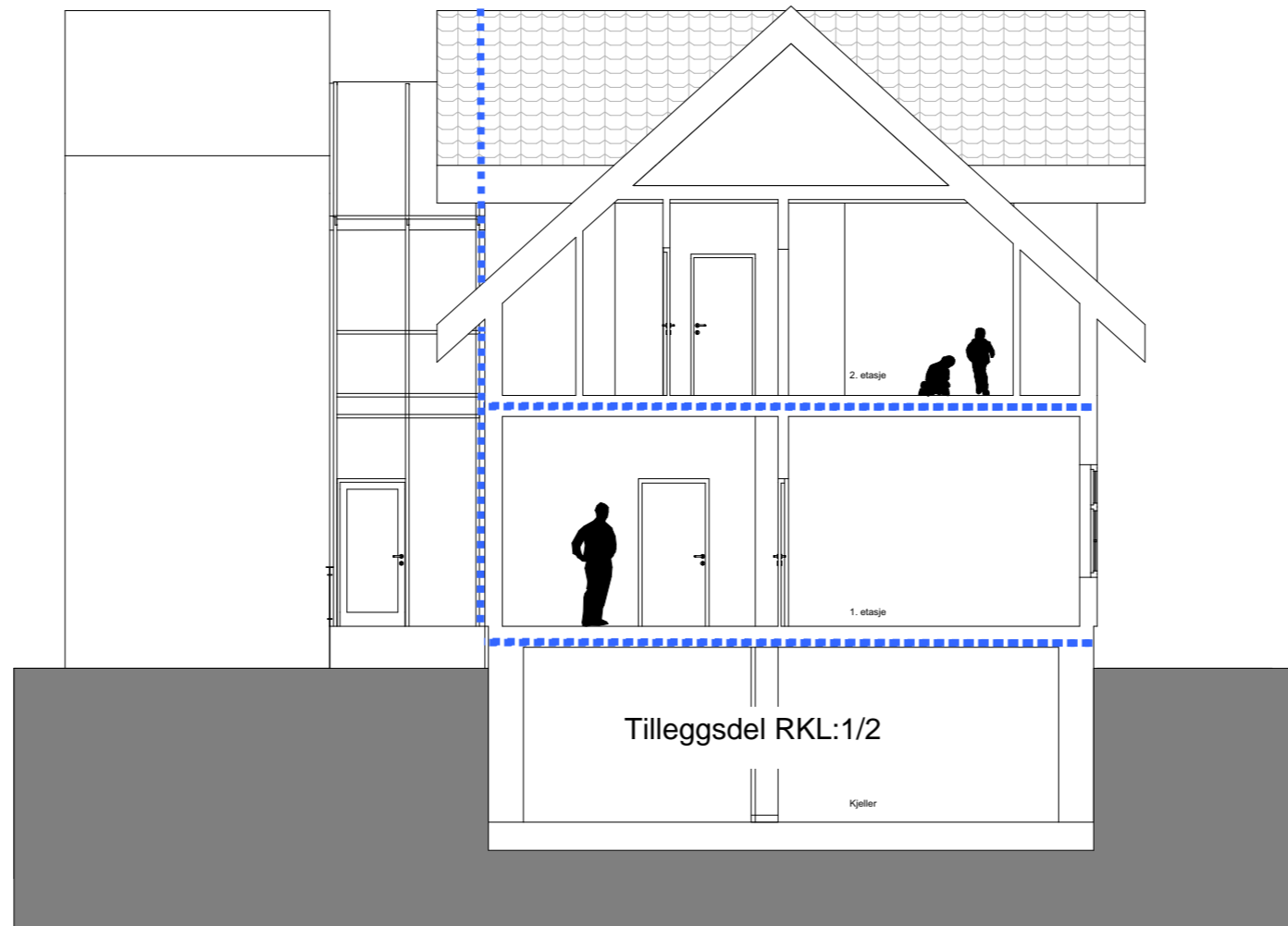
1:100 Snitt A
