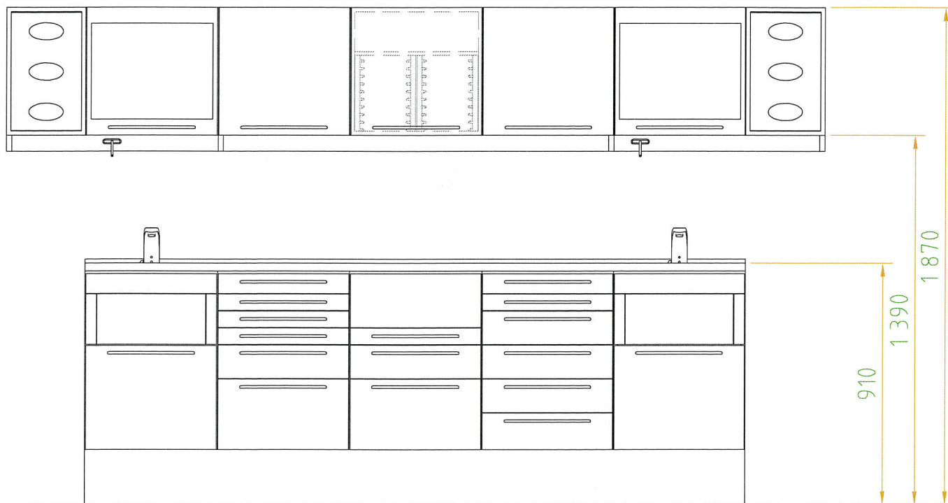
Oppriss A-A
